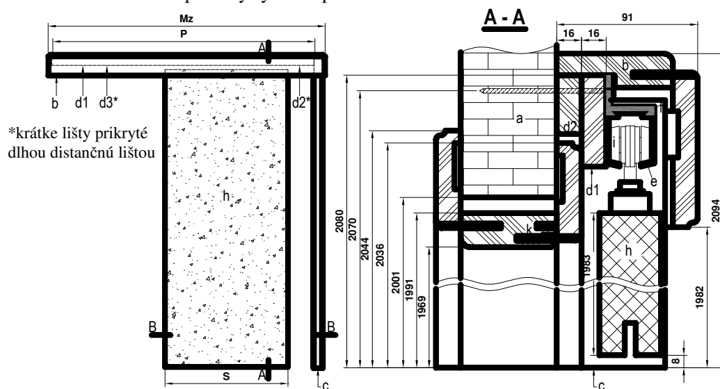
Obr. 4. Pohľad a prierezy systému posuvného NT
