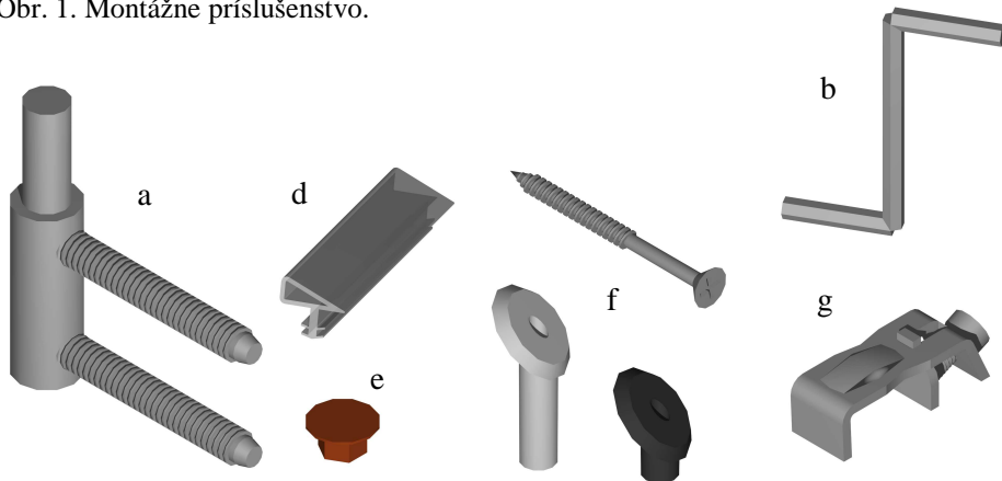
Obr. 1. Montážne príslušenstvo.
