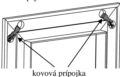
Obr. 7. Spájanie uholníkov
