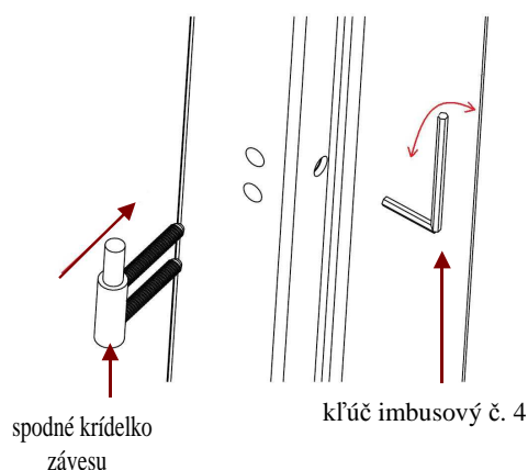
Obr. 4 Montáž závesu
