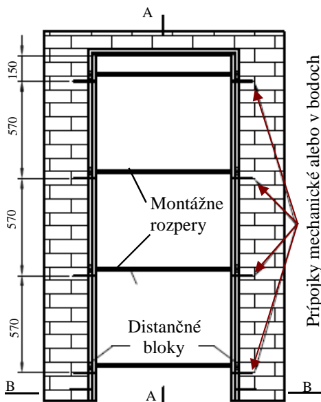
Obr. 9 Montáž zárubni v stene
