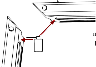
Obr. 7. Spájanie uholníkov
