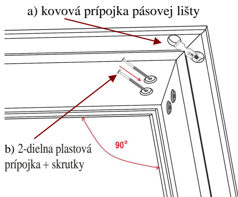
Obr. 3 Spájanie trámov zárubni
